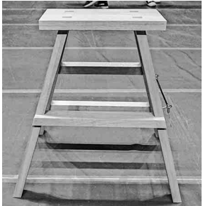
四方転び踏み台
